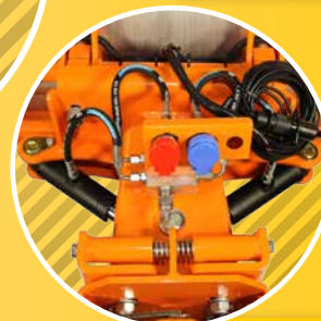
4 HYDR. WINKELVERSTELLUNG HYDR. ANGLE ADJUSTMENT REGLAGE HYDRAULIQUE DE L'ORIENTATION
